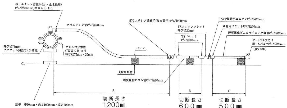
実技課程の給水管配管課題図（全国標準検定）
